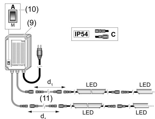
Bild 7: Schutzart IP64 / Anschlussart C
