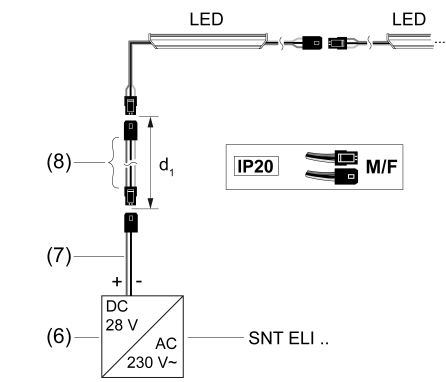
Bild 8: Schutzart IP20 / Anschlussart M/F
