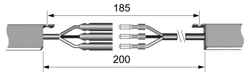
Bild 2: Leuchte montieren
