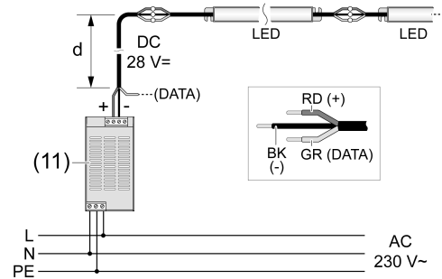
Bild 5: Schaltskizze
