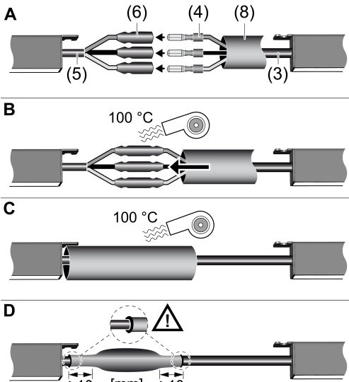
Bild 6: LED-Lampen verketten
