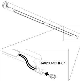
Ausgangsleitung des letzten Lichteinsatzes versiegeln Sealing output cable of the last LED lighting insert
