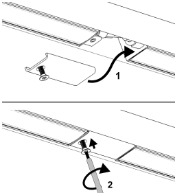
Nutabdeckung montieren Installing groove cover
