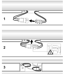
Lichteins a tze verketteten Linking lighting inserts
